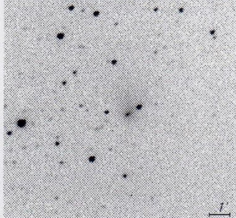
C/1997 T1 (Utsunomiya) Feb. 5, 1998
