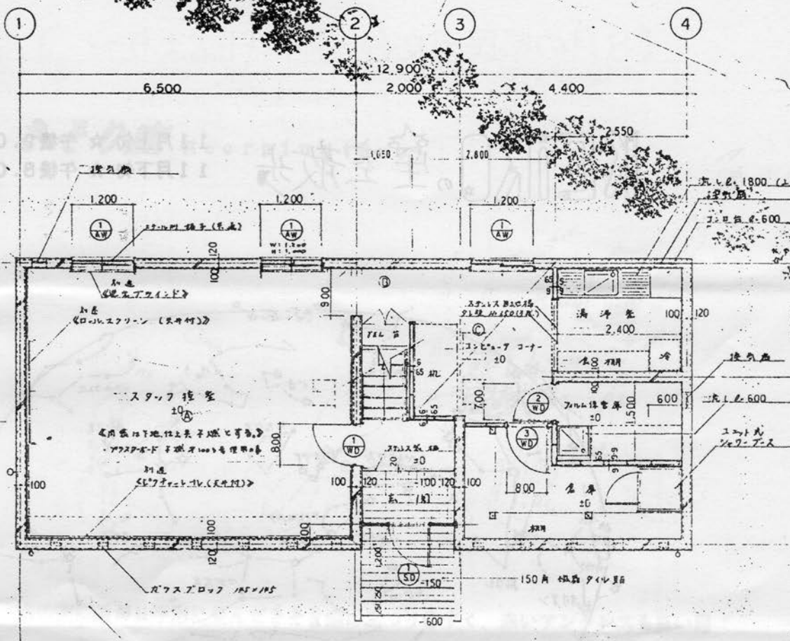
1 階平面図
